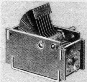
Ein KW-Abstimmkondensator in Aluminium-eifengehäuse. Werkaufnahme KHS.
