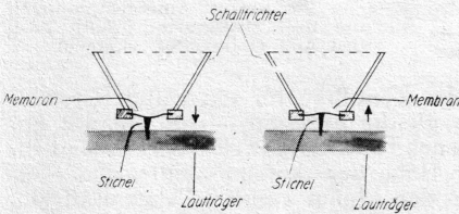
Bild 1. Je nach der Größe der Membrandurchbiegung, d. h. je nach Lautstärke, dringt der Stichel mehr oder weniger tief in die Wachsfläche. So entsteht die Tiefenschrift. (Edisonschrift).
