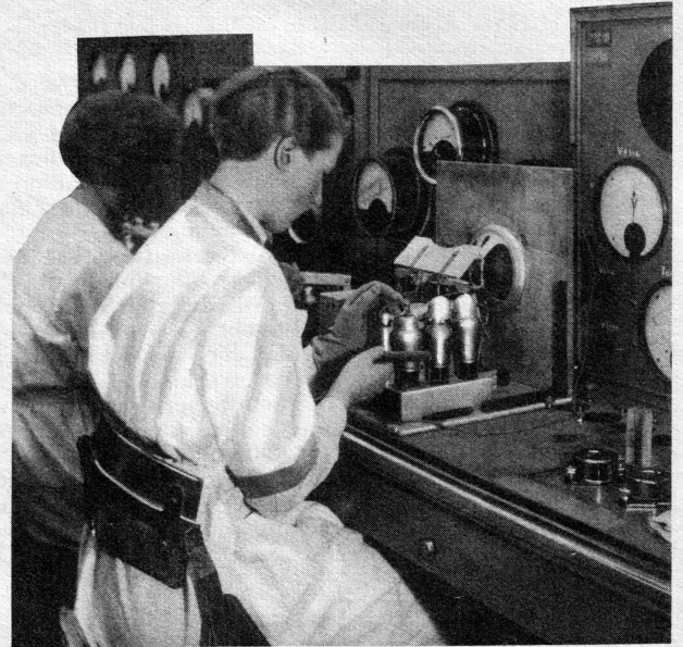
Eine der vielen, vielen Prüfungen, die jede Röhre zu bestehen hat: Die Klopfprüfung mit einem Gummitast, die zeigen soll, ob die Röhre Kratzen, Krachen oder Brummen verursacht.
