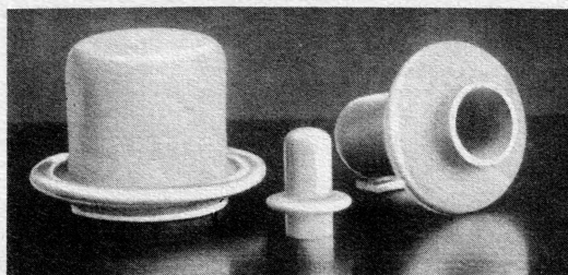
Ein Sendeblock in Topfform für hohe Spannungen und große Wertgenauigkeit. Aufn. Hefcho.
