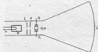
Abb. 1a. Schnitt durch eine Braunische Röhre. H: Heizfaden oder Kathode, W: Wehneltzylinder, L: Linse, A: Anode, P 1 P 1 : Ablenkplattenpaare, P 2 P 2 : Ablenkplattenpaare, L c : Leuchtschirm.
