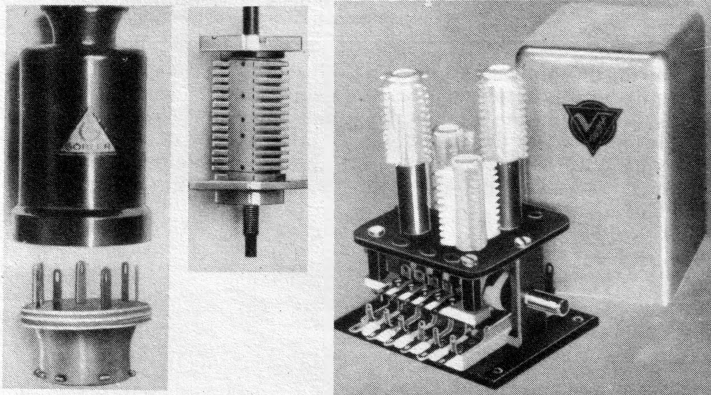
Eine Kurzwellensteckspule mit Eisenkern, wobei als Fassung jede Röhrenfassung verwendet werden kann. Das Bild zeigt den Sockel, die Hülse und den Wickelkörper. Verkaufnahme Görler.
