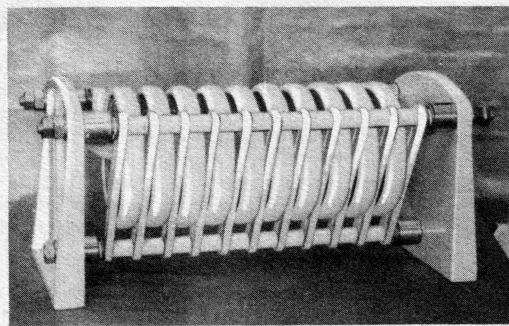
Ein Hochleistungsblockkondensator aus feuerverfilberten Caliteinzelelementen. Die Einzelelemente sind einfach hintereinander angeordnet, und entsprechend zusammengefasst. Werkaufnahme Hefcho.
