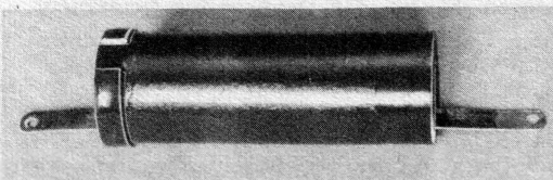
Ein Rohrkondensator aus Calit und Kondensa, wie er für Kleinfender oft gebraucht wird. Werkaufnahme Hefcho.
